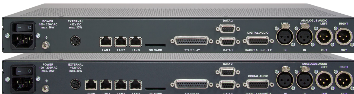
MAGIC ACip3 (oben) und MAGIC ACip3 2M (unten) MAGIC ACip3 2M verfügt über eine E1-Schnittstelle und ist nur auf Anfrage erhältlich
